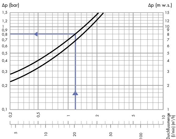
Diagramm 2 (Druckabfall)
